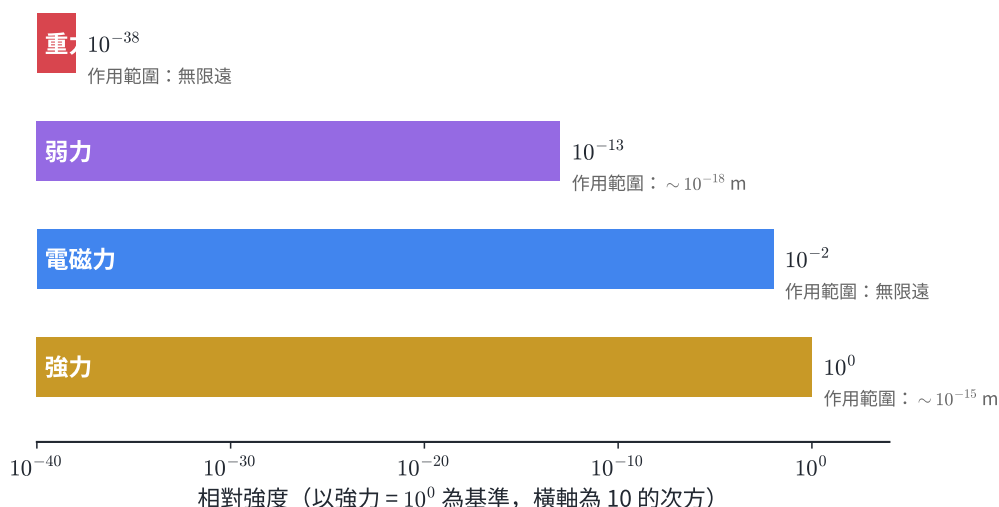
圖 3-4：四種基本交互作用的相對強度（以強力為 1，橫軸為 10 的次方）。四者強度差距極大，從強力的 1 到重力的約 10^{-38} 。圖中同時標出各力的作用範圍。
